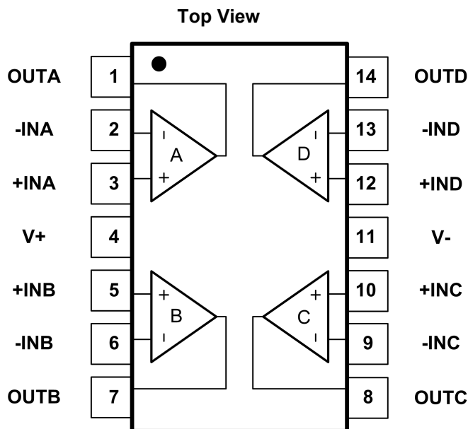
Fig.4-3. GT8444: PD(SOP14) Package GT8444: TD(TSSOP14) Package
