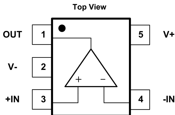
Fig.4-1. GT8441: S5(SOT23-5) Package
