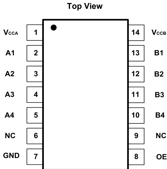
Fig.4-3. GT0104: TD (TSSOP14) Package
