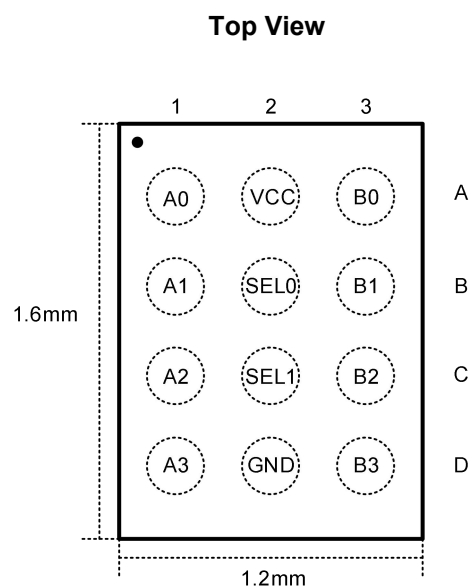
Fig.4-1.GT550: WLG (WLCSP-12L) Package
