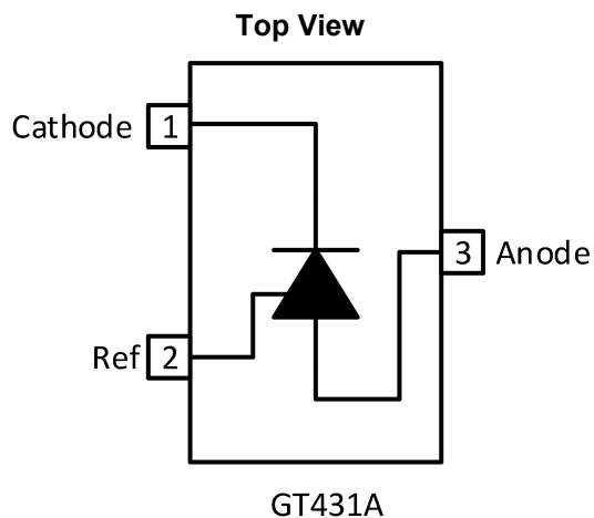
Fig.5-1. GT431A: SOT23(3) Package
