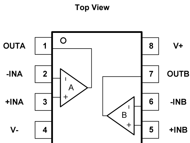
Fig.5-4. GT722: M8(MSOP8) Package
