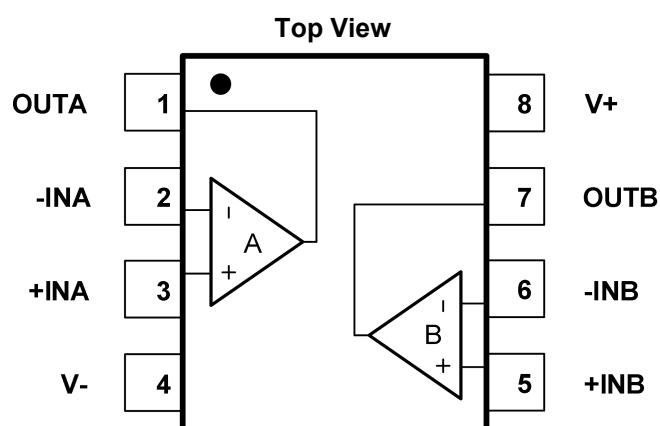
Fig.5-3. GT8952: M8(MSOP8) Package
