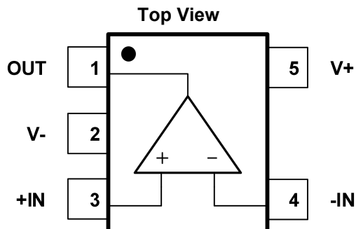
Fig.5-2. GT8951: BC5(SC70-5) Package
