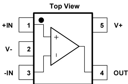
Fig.5-1. GT8951: C5(SC70-5) Package
