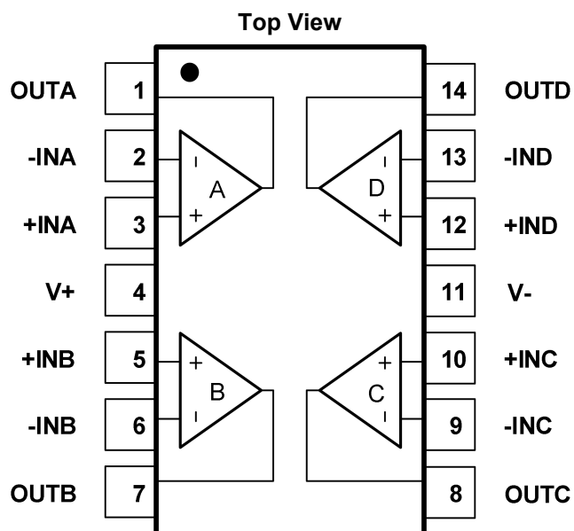
Fig.5-4. GT8954: TD(TSSOP14) Package
